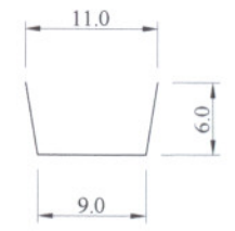
Lateral Groove (2:1 scale)
