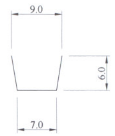
Circ Groove (2:1 scale)
